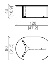
TAVOLINO - COFFEE TABLE 80X120XH43
