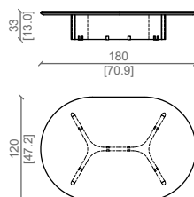
TAVOLINO - COFFEE TABLE 120X180
