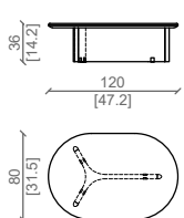
TAVOLINO - COFFEE TABLE 80X120XH36
